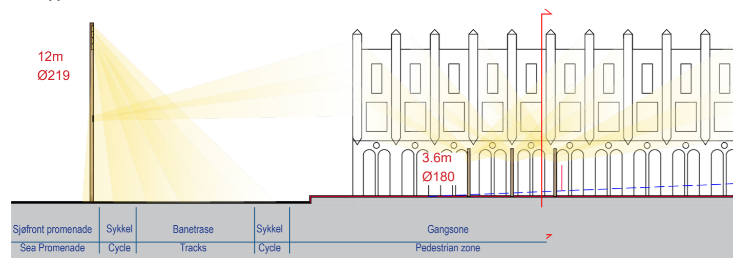
Prinsippsnitt A-A
