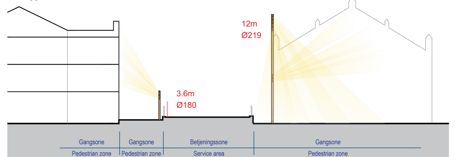
Prinsippsnitt B-B
